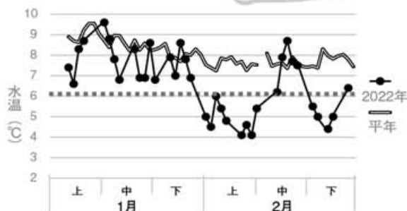
図1 沿岸水温の推移(1~2月、加茂港表層水温)
